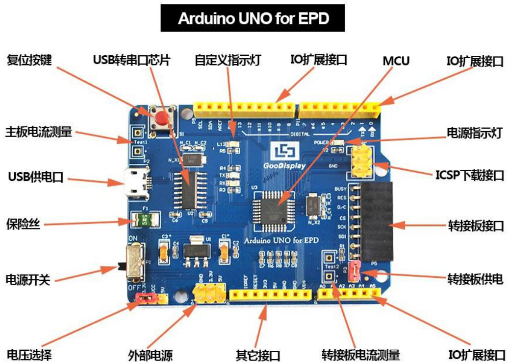
图 1 主板 Arduino UNO for EPD 功能图
