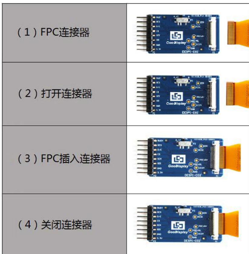
图 4 电子纸与转接板连接方式
